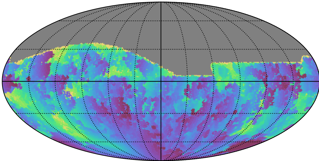
roman_v3.3_10yrs All sky g band: Min solarElong
