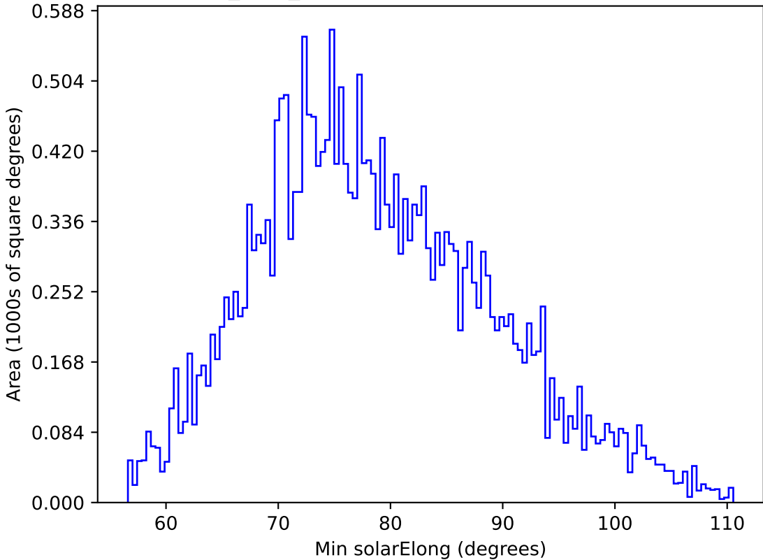
roman_v3.3_10yrs All sky g band: Min solarElong
