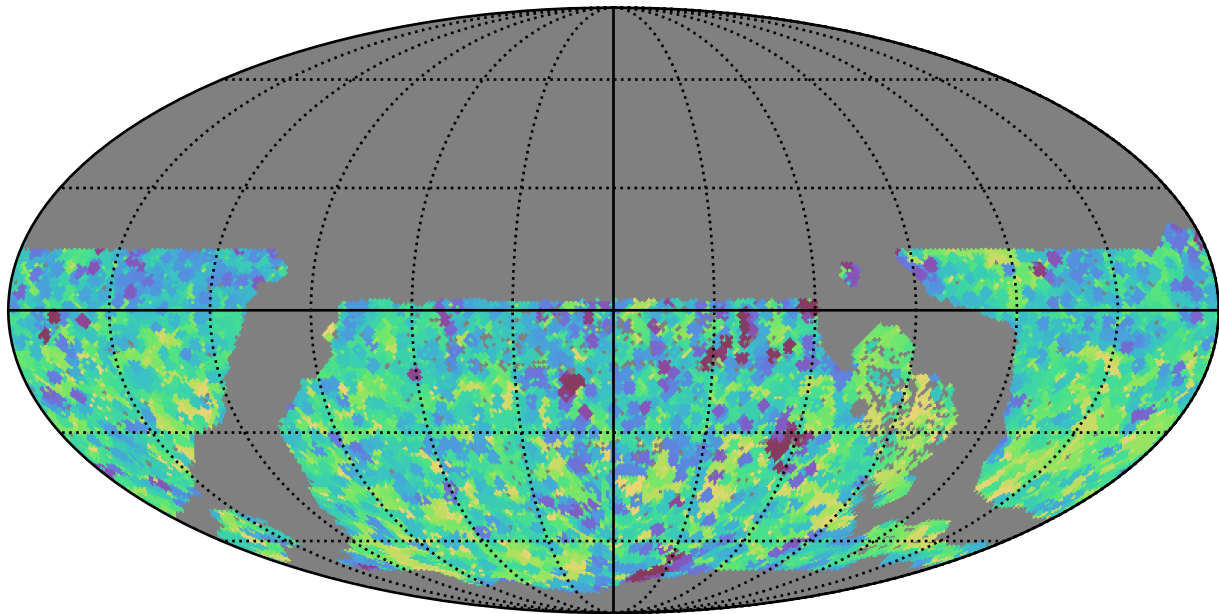
roman_v3.3_10yrs WFD y band: Min skyBrightness
