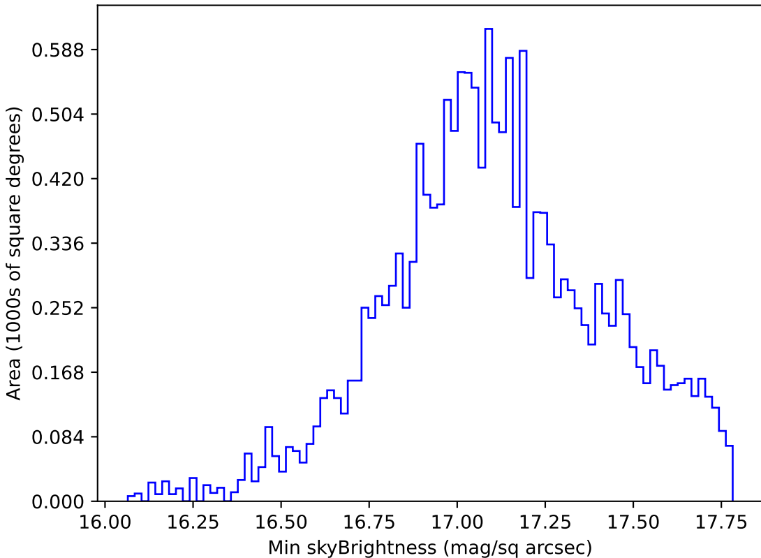
roman_v3.3_10yrs WFD y band: Min skyBrightness
