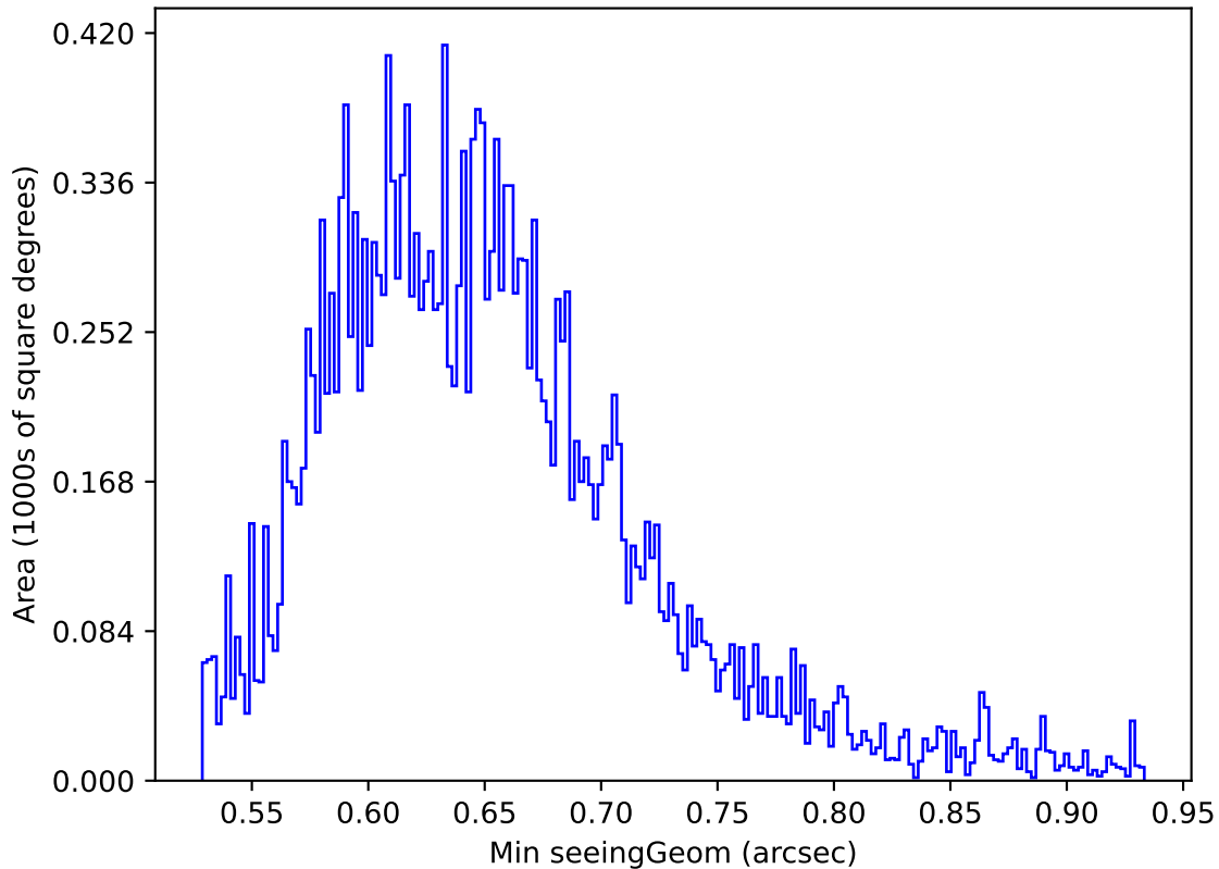
roman_v3.3_10yrs Yr 1 y band: Min seeingGeom
