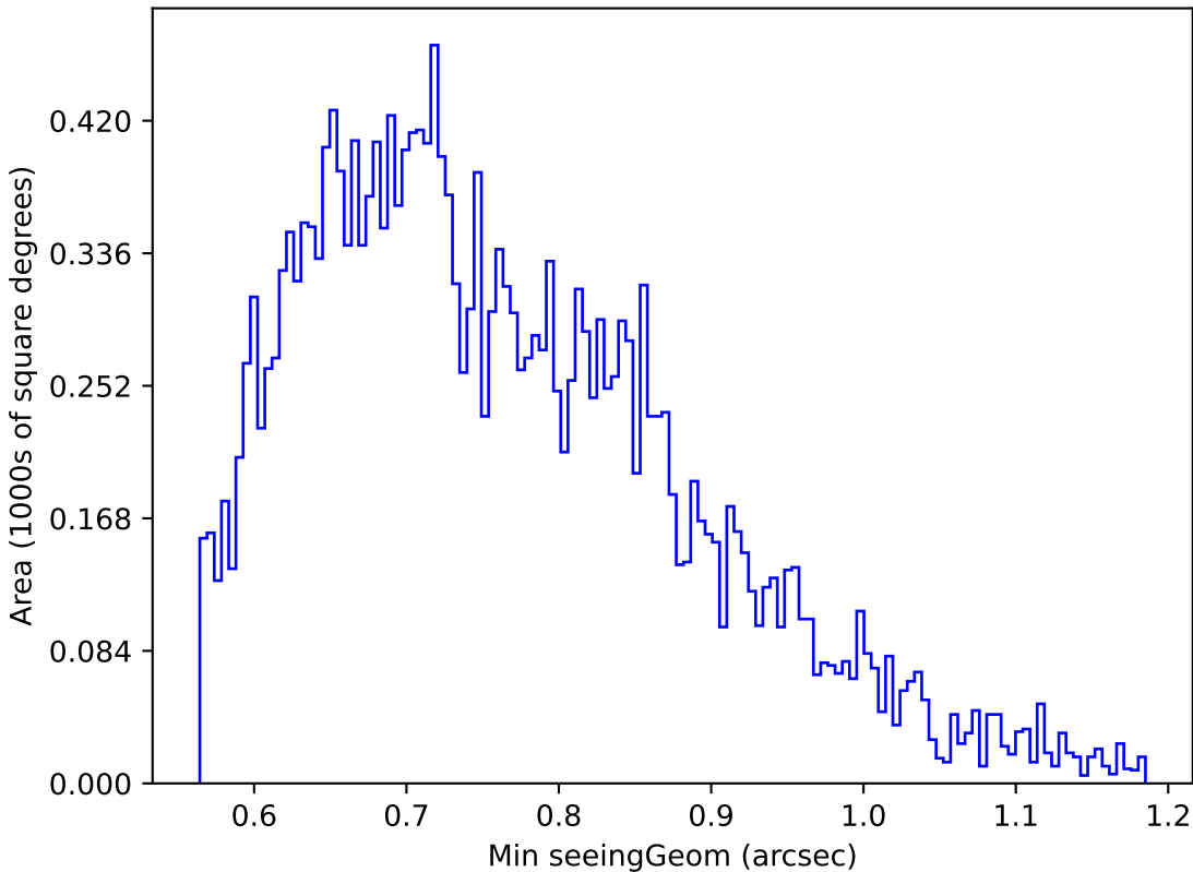
roman_v3.3_10yrs Yr 1 u band: Min seeingGeom
