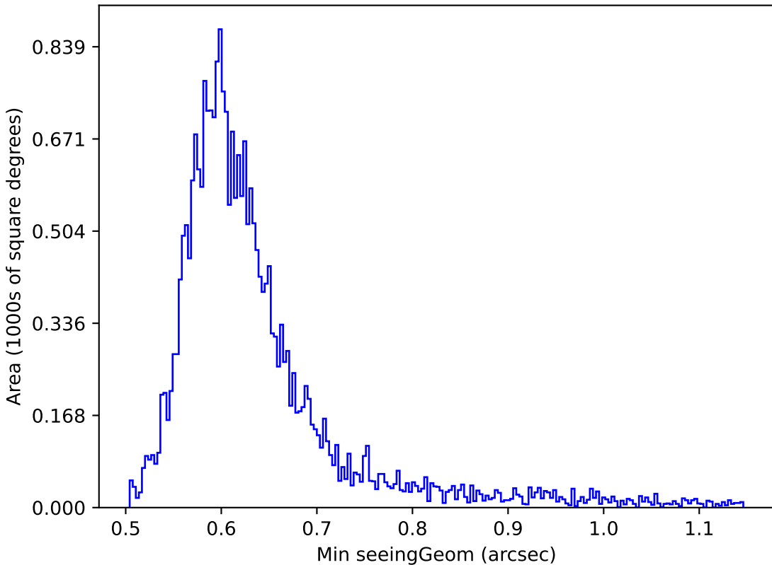
roman_v3.3_10yrs Yr 1 r band: Min seeingGeom
