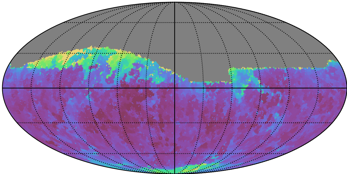
roman_v3.3_10yrs Yr 1 i band: Min seeingGeom
