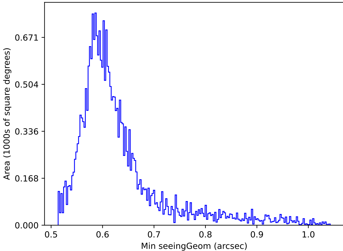
roman_v3.3_10yrs Yr 1 i band: Min seeingGeom
