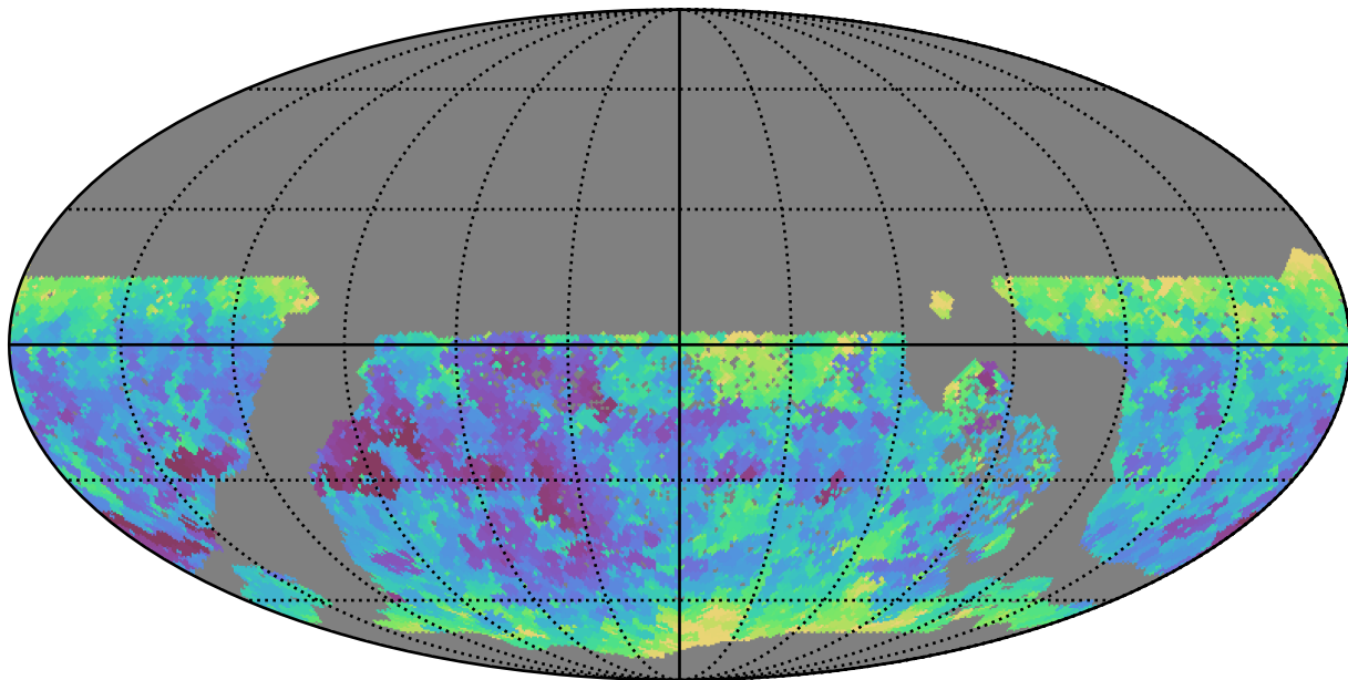
roman_v3.3_10yrs WFD y band: Min seeingEff
