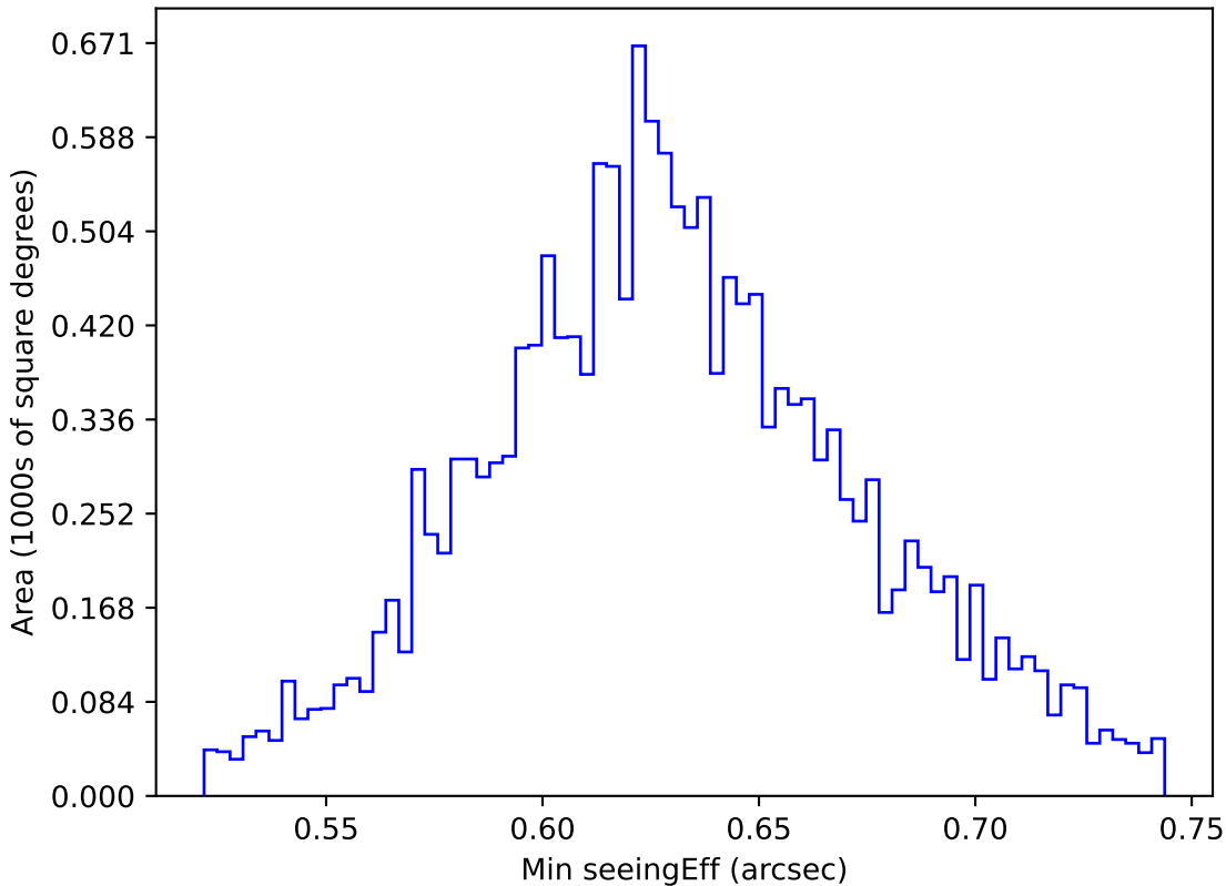
roman_v3.3_10yrs WFD y band: Min seeingEff
