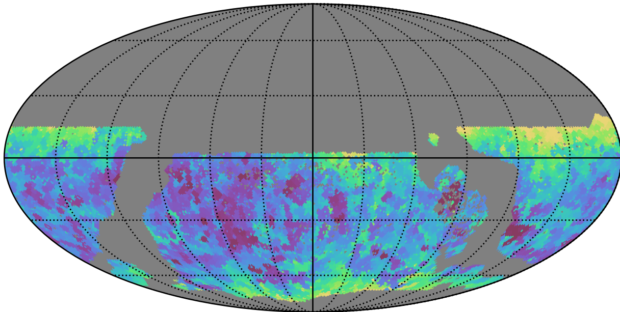
roman_v3.3_10yrs WFD i band: Min seeingEff
