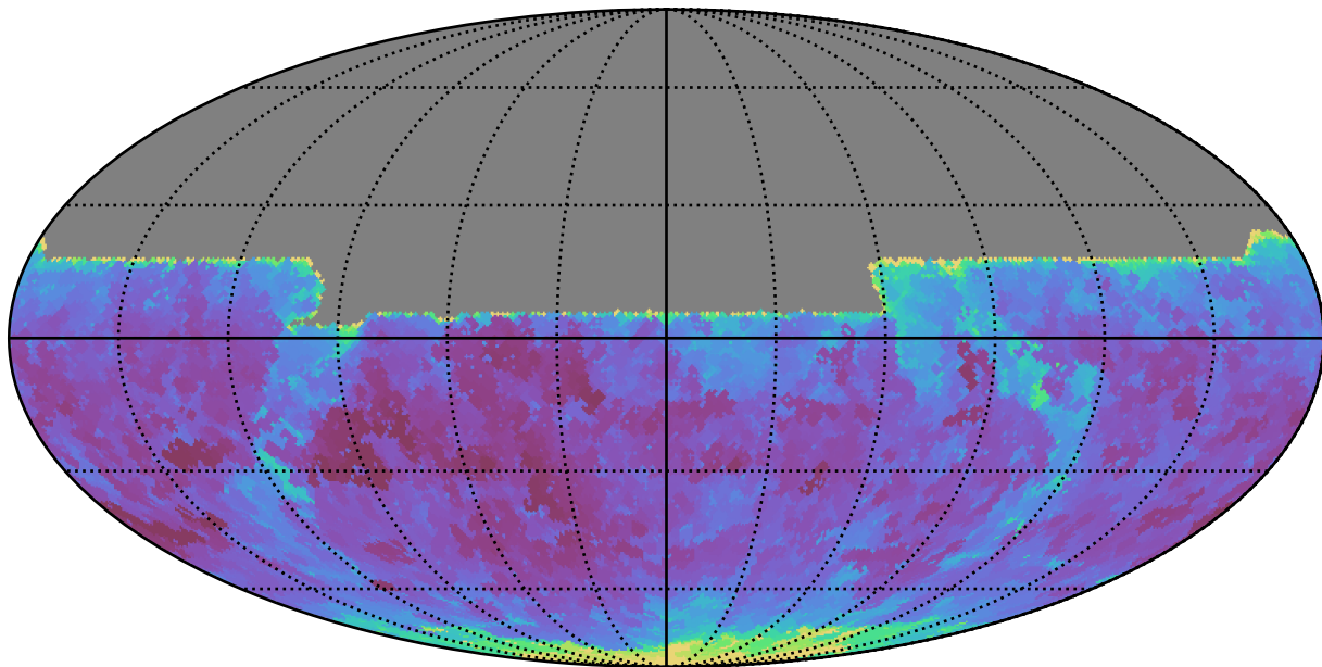
roman_v3.3_10yrs All sky y band: Min seeingEff
