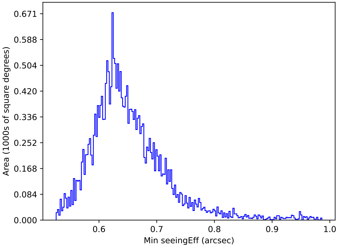
roman_v3.3_10yrs All sky y band: Min seeingEff
