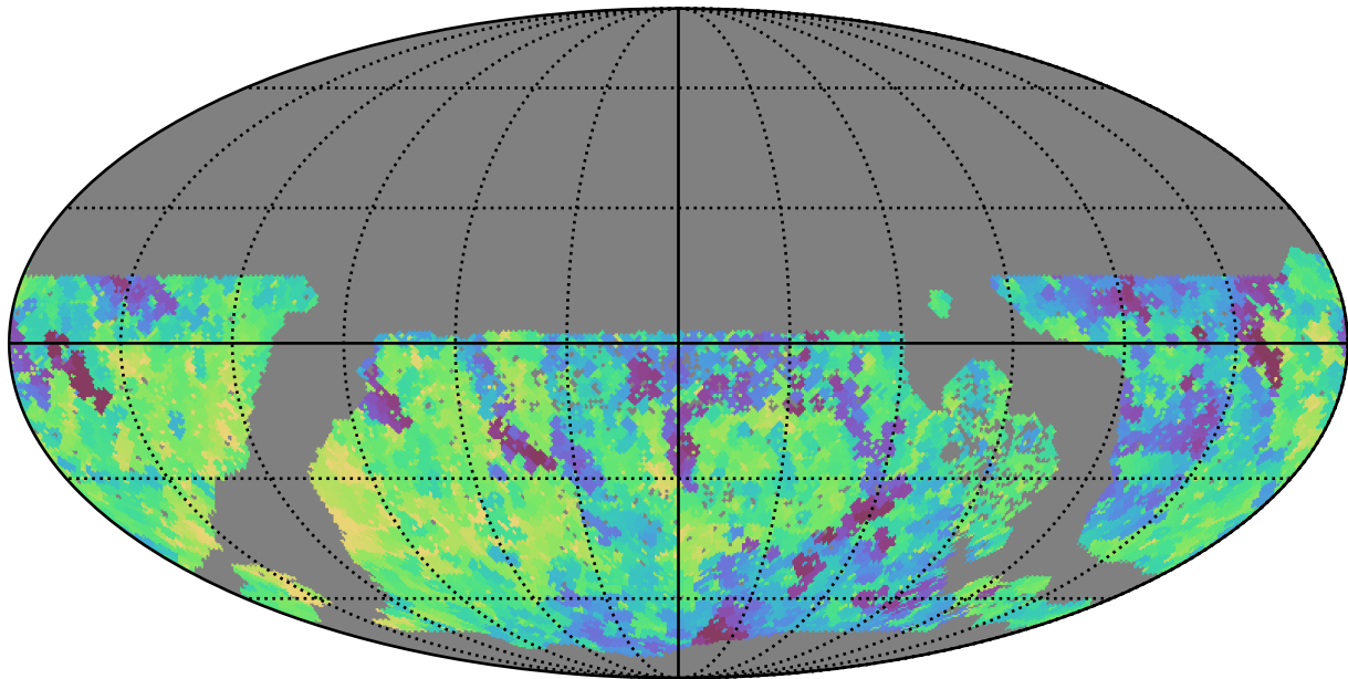
roman_v3.3_10yrs WFD z band: Min saturation_mag
