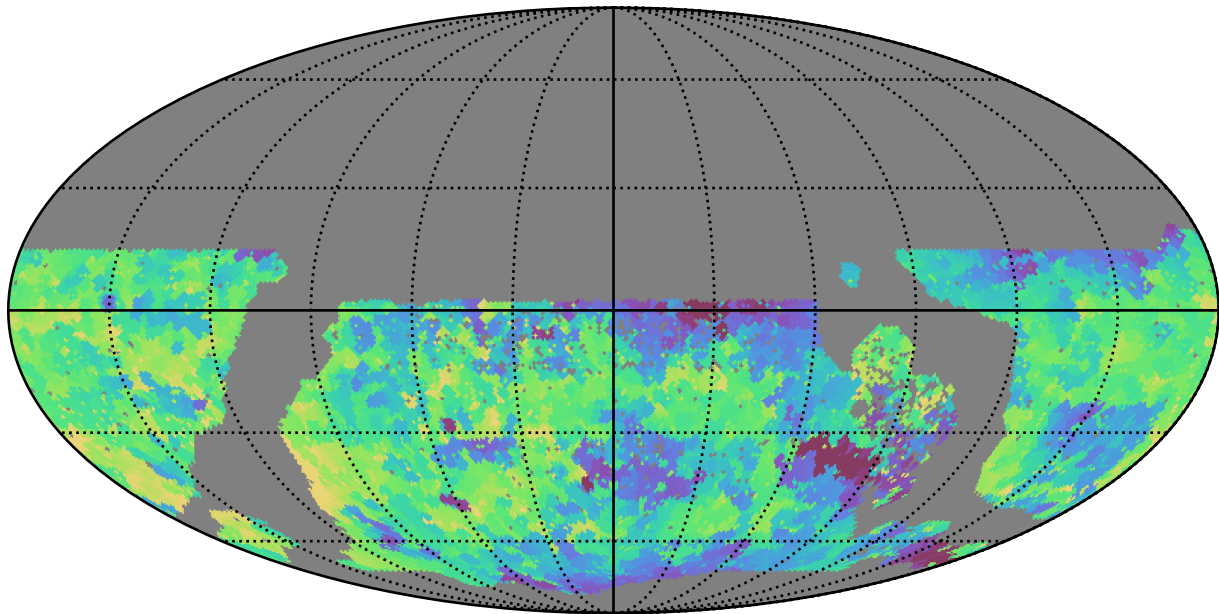
roman_v3.3_10yrs WFD u band: Min saturation_mag
