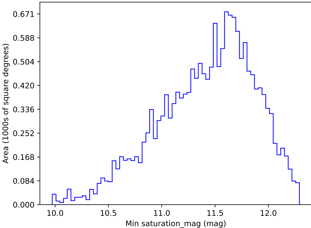
roman_v3.3_10yrs WFD u band: Min saturation_mag
