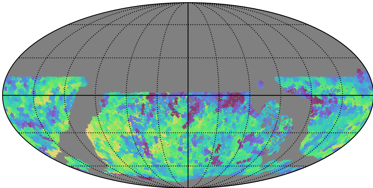
roman_v3.3_10yrs WFD r band: Min saturation_mag
