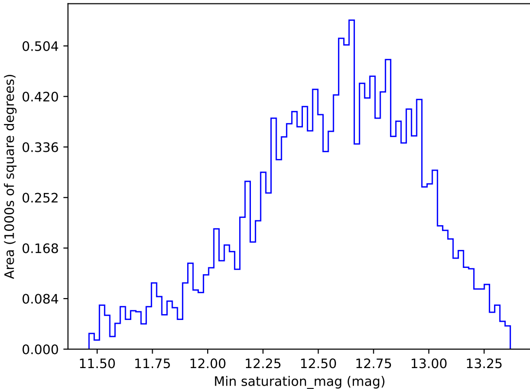
roman_v3.3_10yrs WFD r band: Min saturation_mag
