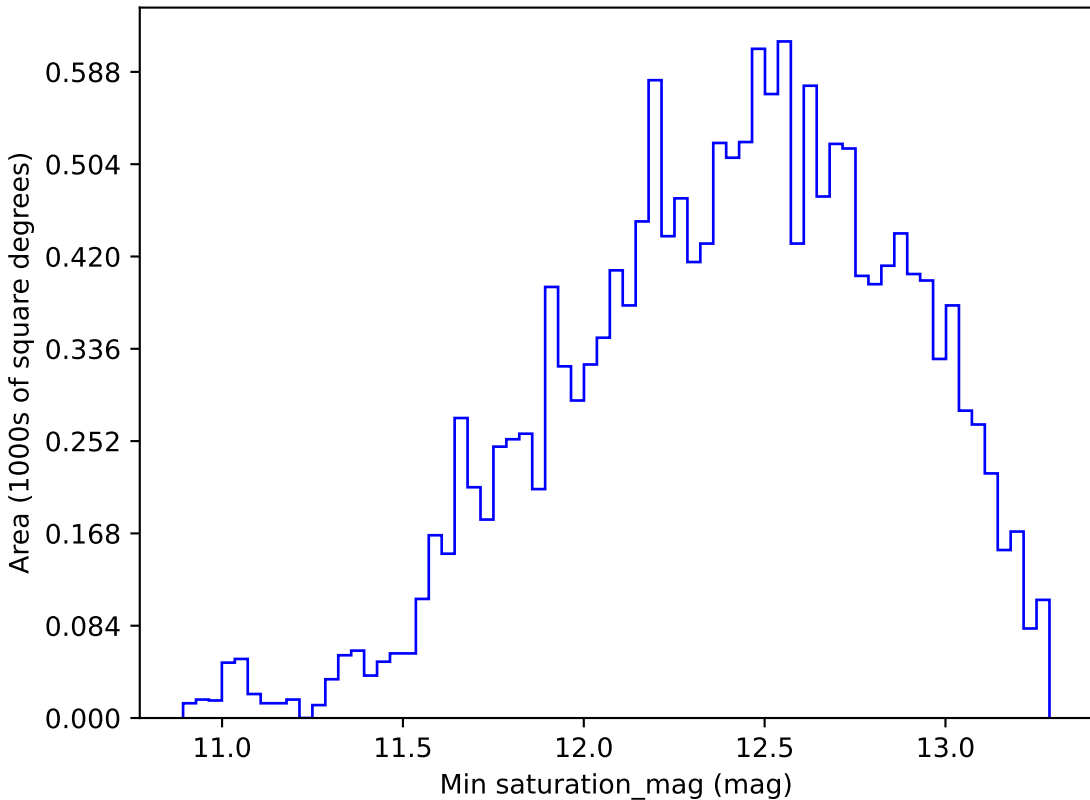
roman_v3.3_10yrs WFD i band: Min saturation_mag
