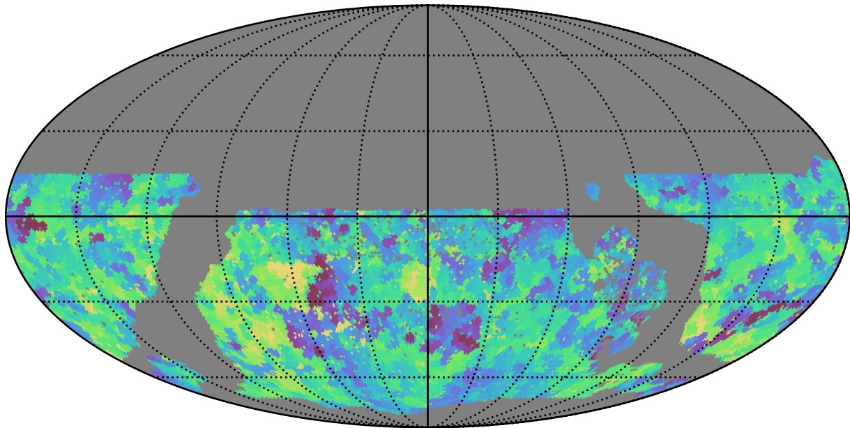
roman_v3.3_10yrs WFD g band: Min saturation_mag
