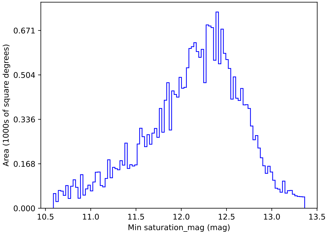
roman_v3.3_10yrs All sky z band: Min saturation_mag
