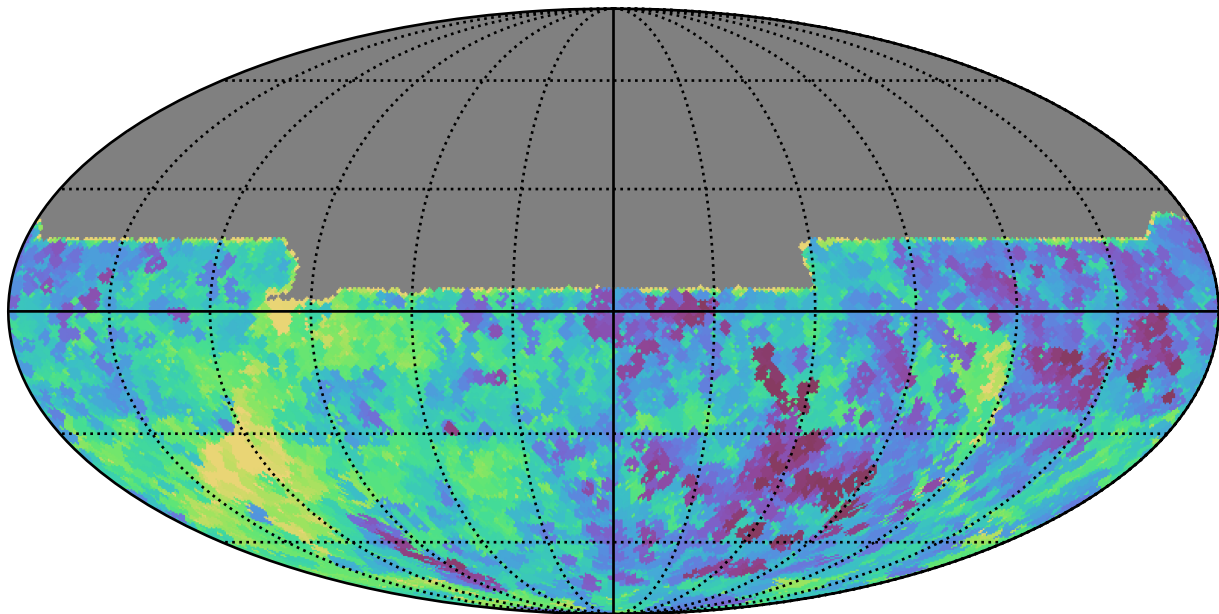
roman_v3.3_10yrs All sky y band: Min saturation_mag
