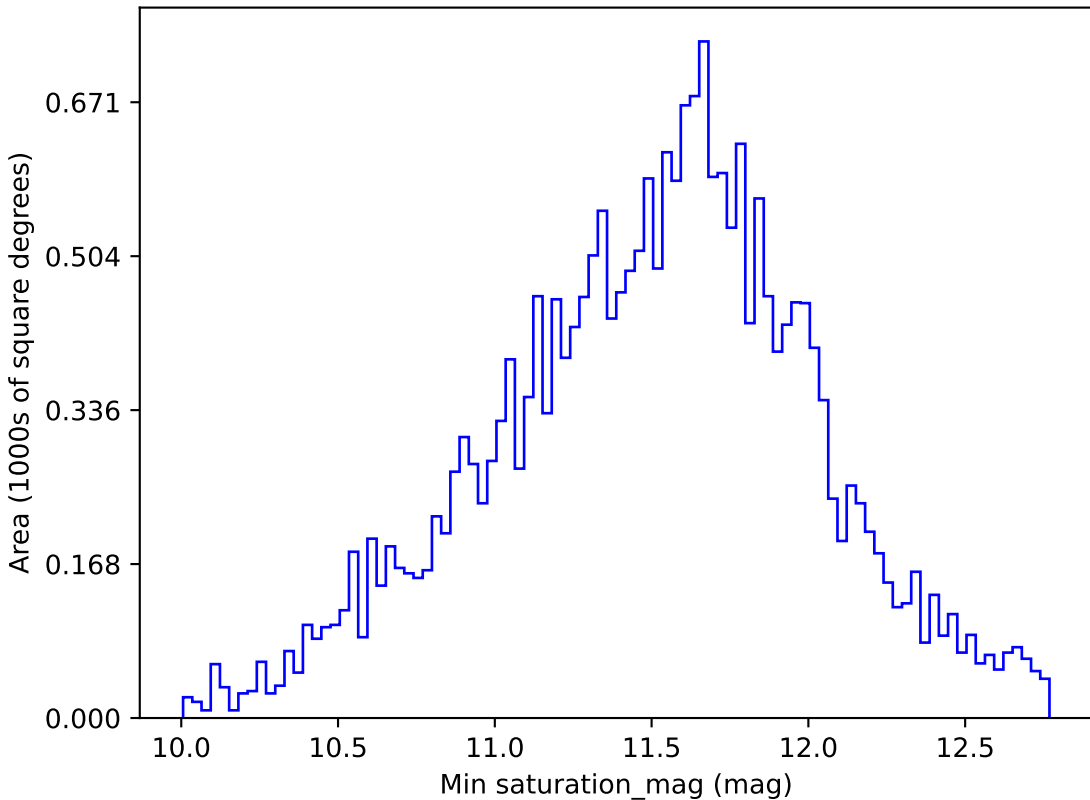
roman_v3.3_10yrs All sky u band: Min saturation_mag
