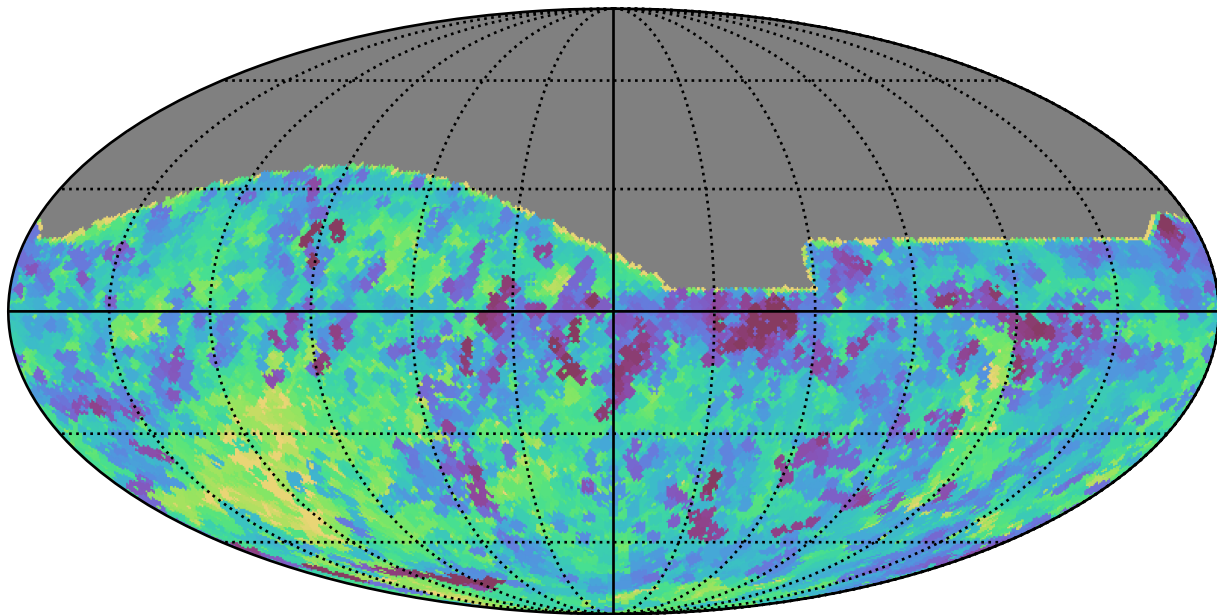
roman_v3.3_10yrs All sky r band: Min saturation_mag
