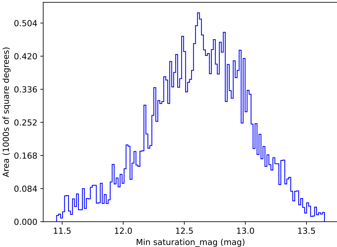
roman_v3.3_10yrs All sky r band: Min saturation_mag
