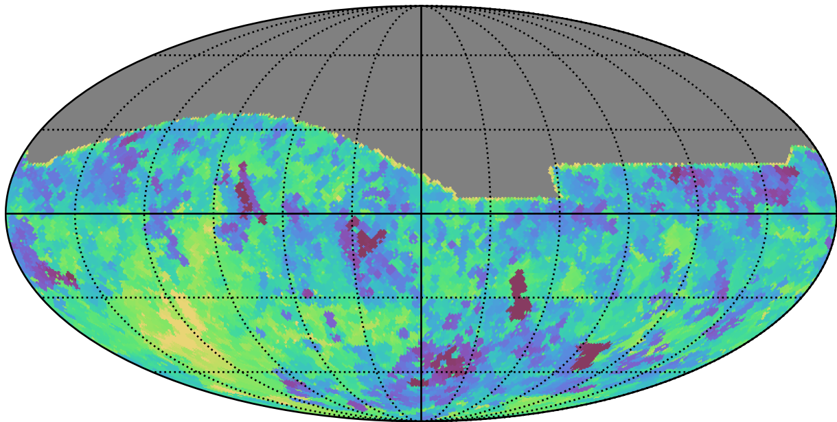
roman_v3.3_10yrs All sky i band: Min saturation_mag
