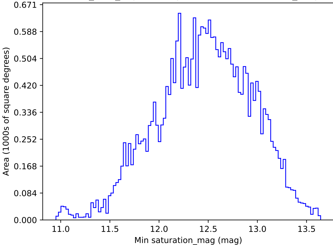
roman_v3.3_10yrs All sky i band: Min saturation_mag
