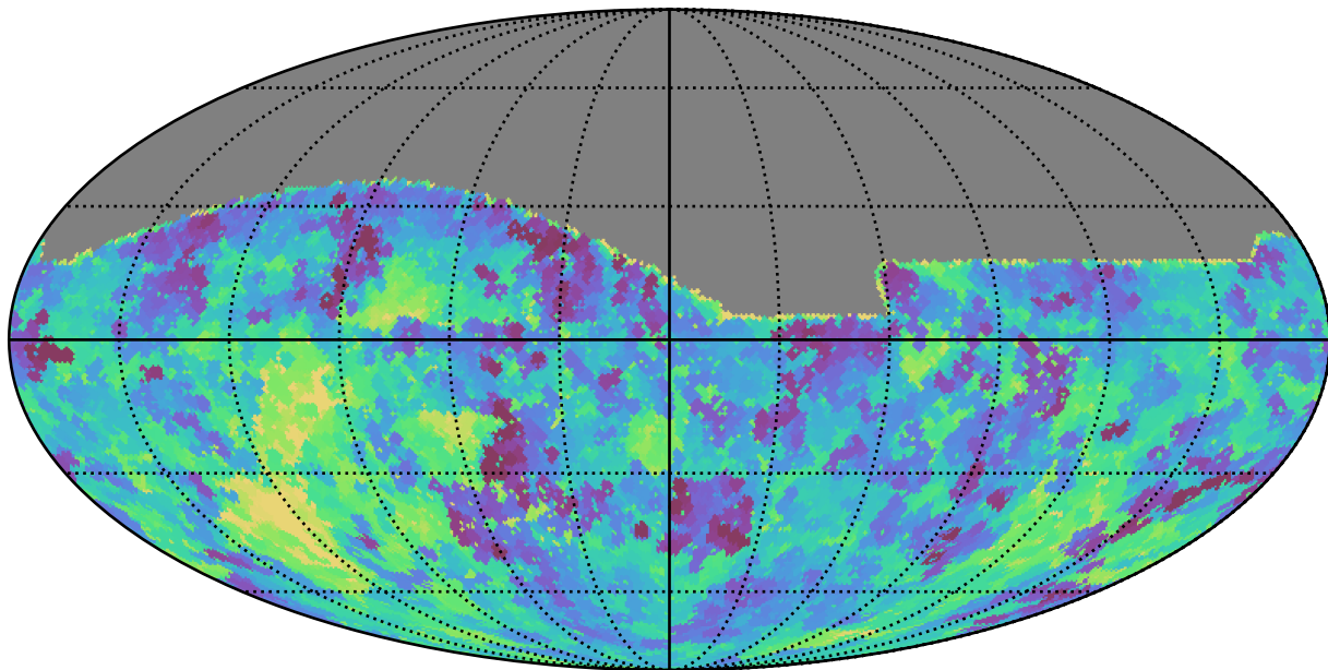
roman_v3.3_10yrs All sky g band: Min saturation_mag
