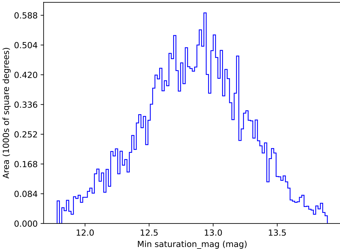
roman_v3.3_10yrs All sky g band: Min saturation_mag
