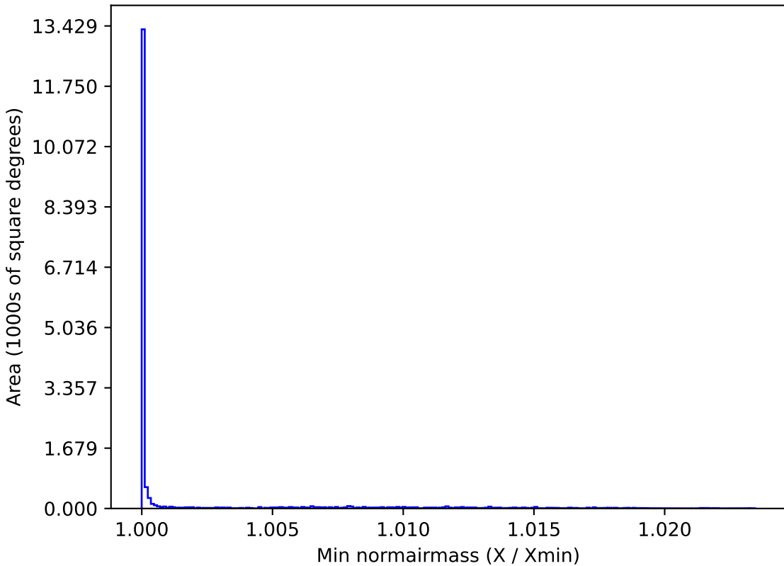
roman_v3.3_10yrs WFD z band: Min normairmass
