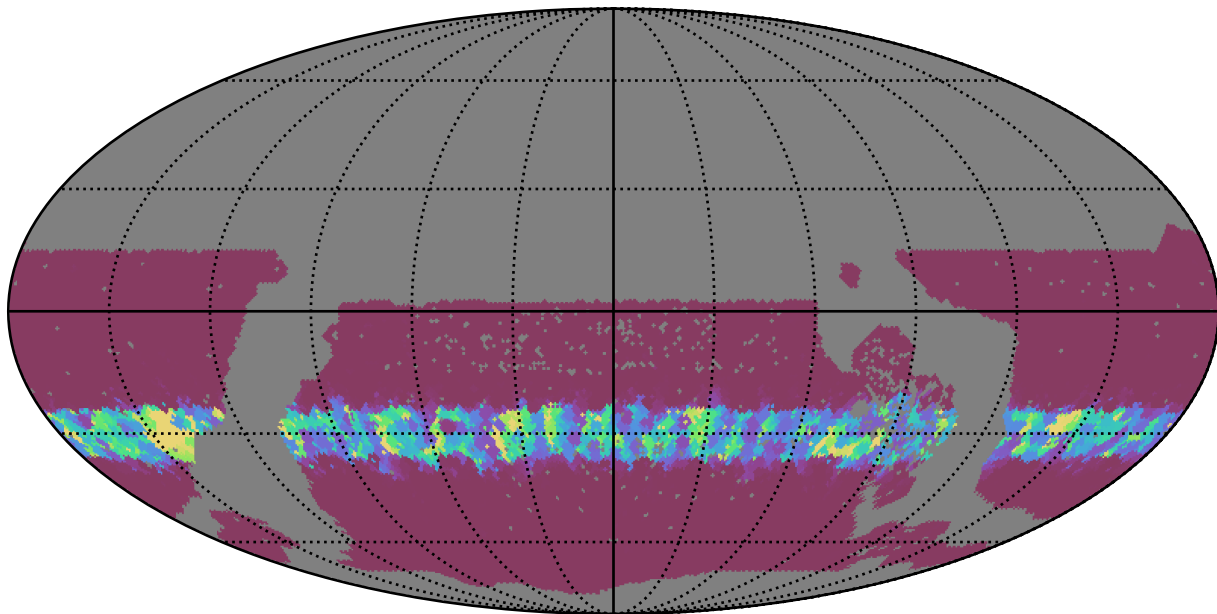
roman_v3.3_10yrs WFD y band: Min normairmass
