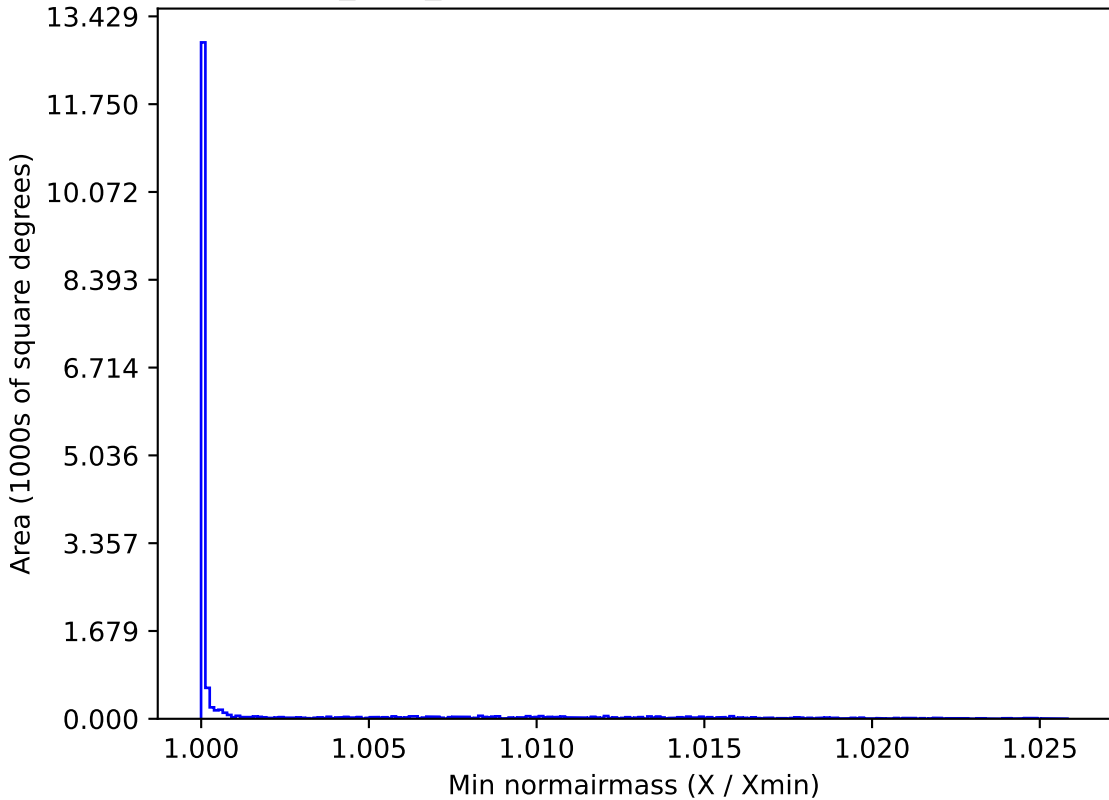
roman_v3.3_10yrs WFD y band: Min normairmass
