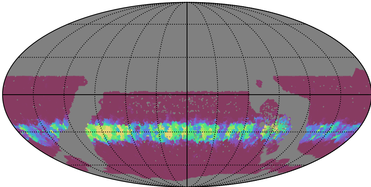
roman_v3.3_10yrs WFD u band: Min normairmass
