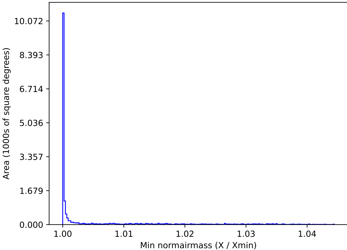
roman_v3.3_10yrs WFD u band: Min normairmass
