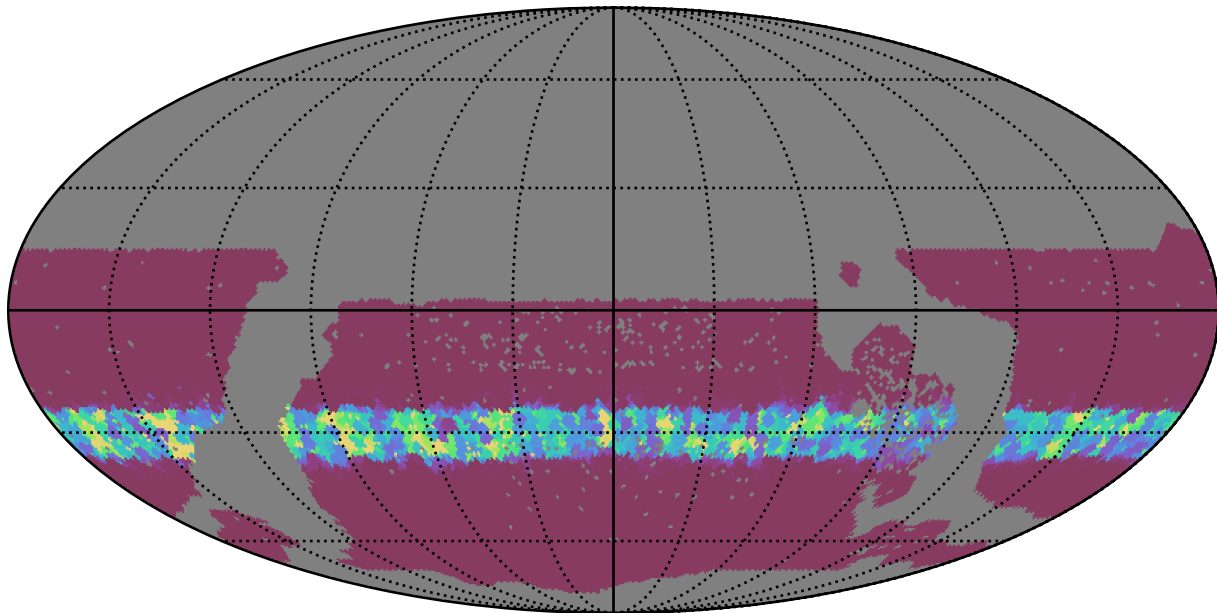
roman_v3.3_10yrs WFD r band: Min normairmass
