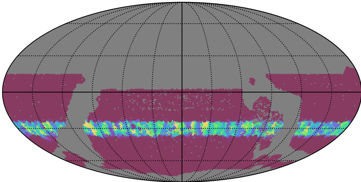
roman_v3.3_10yrs WFD i band: Min normairmass
