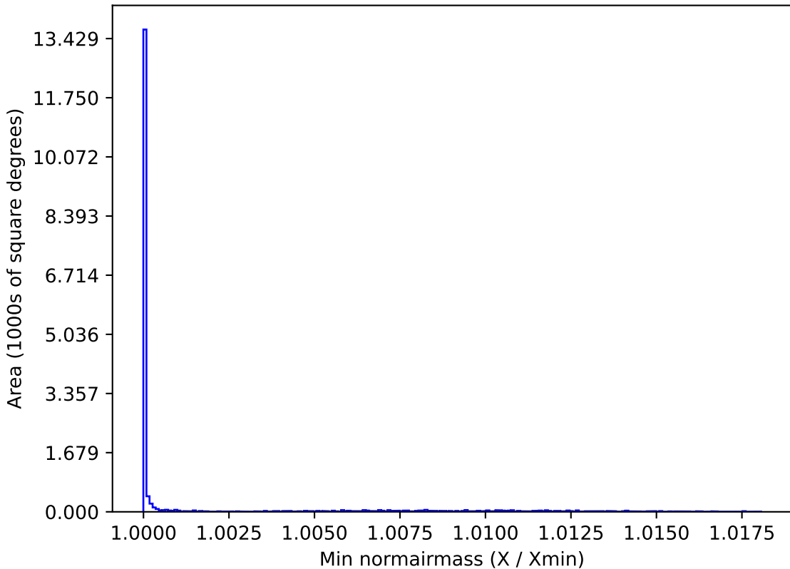
roman_v3.3_10yrs WFD i band: Min normairmass
