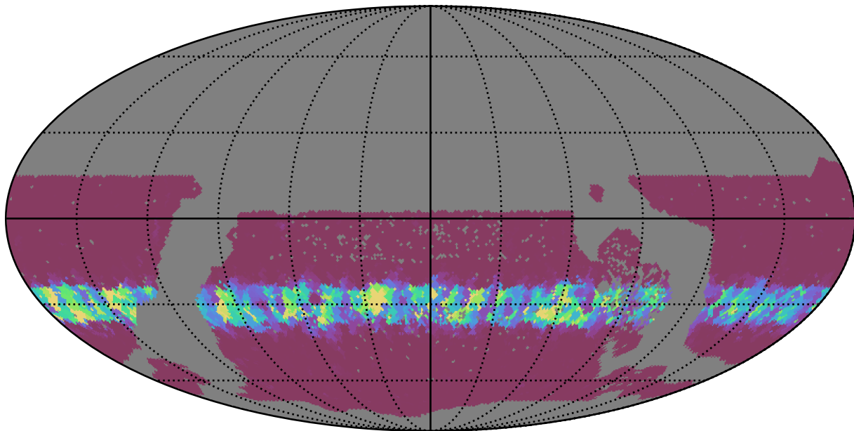
roman_v3.3_10yrs WFD g band: Min normairmass
