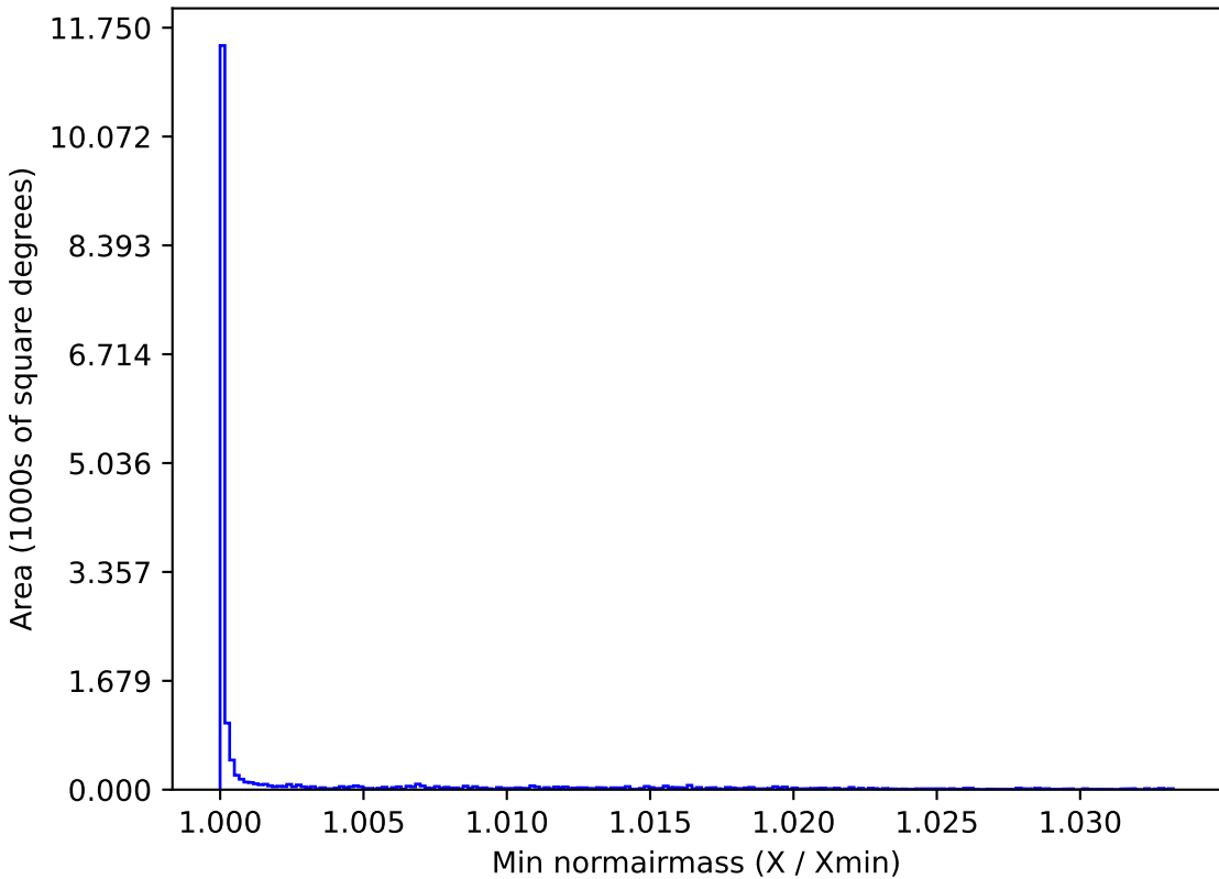
roman_v3.3_10yrs WFD g band: Min normairmass
