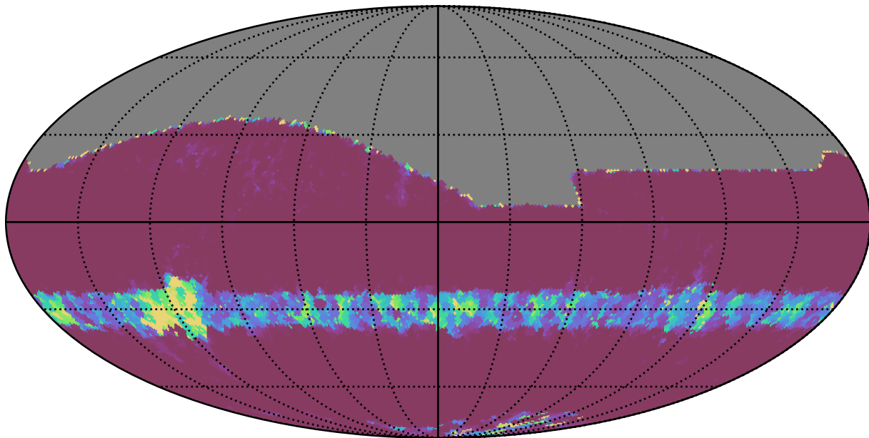
roman_v3.3_10yrs All sky z band: Min normairmass
