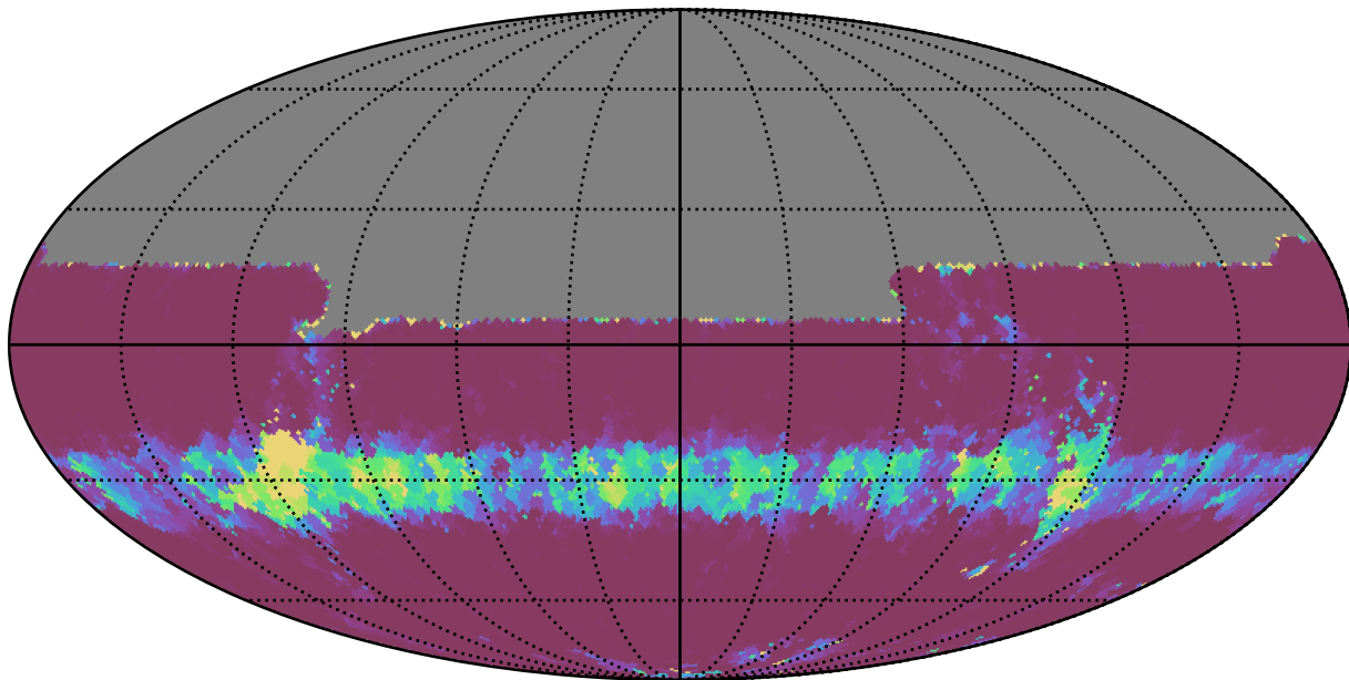
roman_v3.3_10yrs All sky u band: Min normairmass
