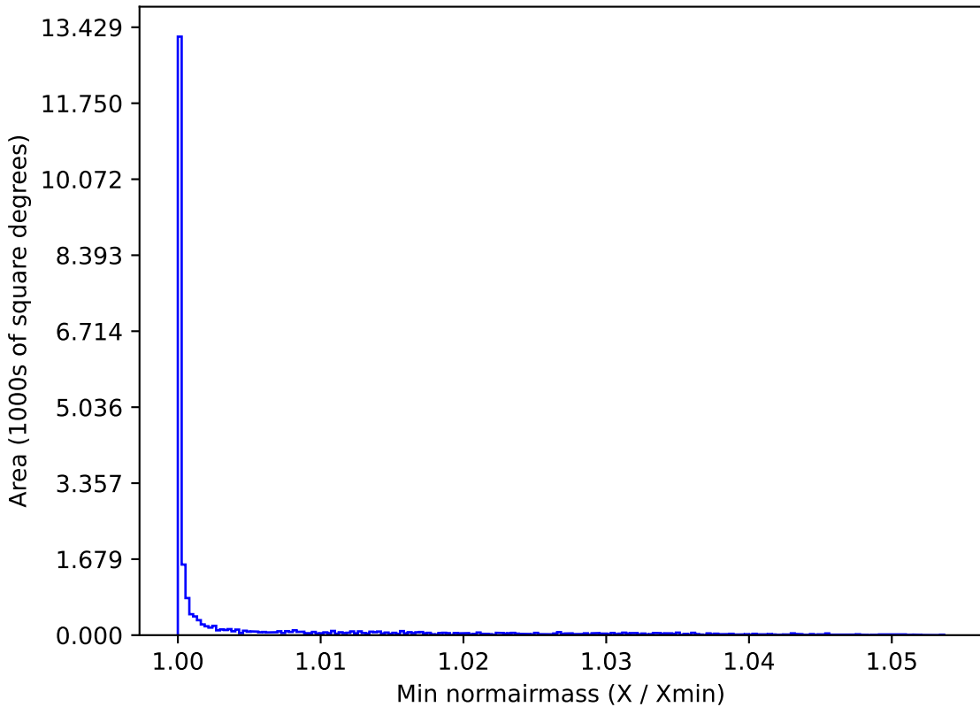
roman_v3.3_10yrs All sky u band: Min normairmass
