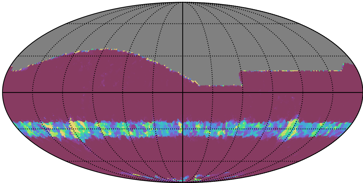
roman_v3.3_10yrs All sky r band: Min normairmass
