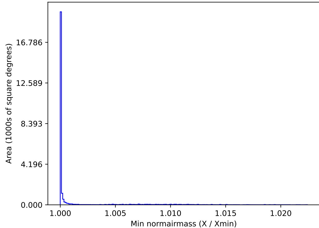
roman_v3.3_10yrs All sky r band: Min normairmass
