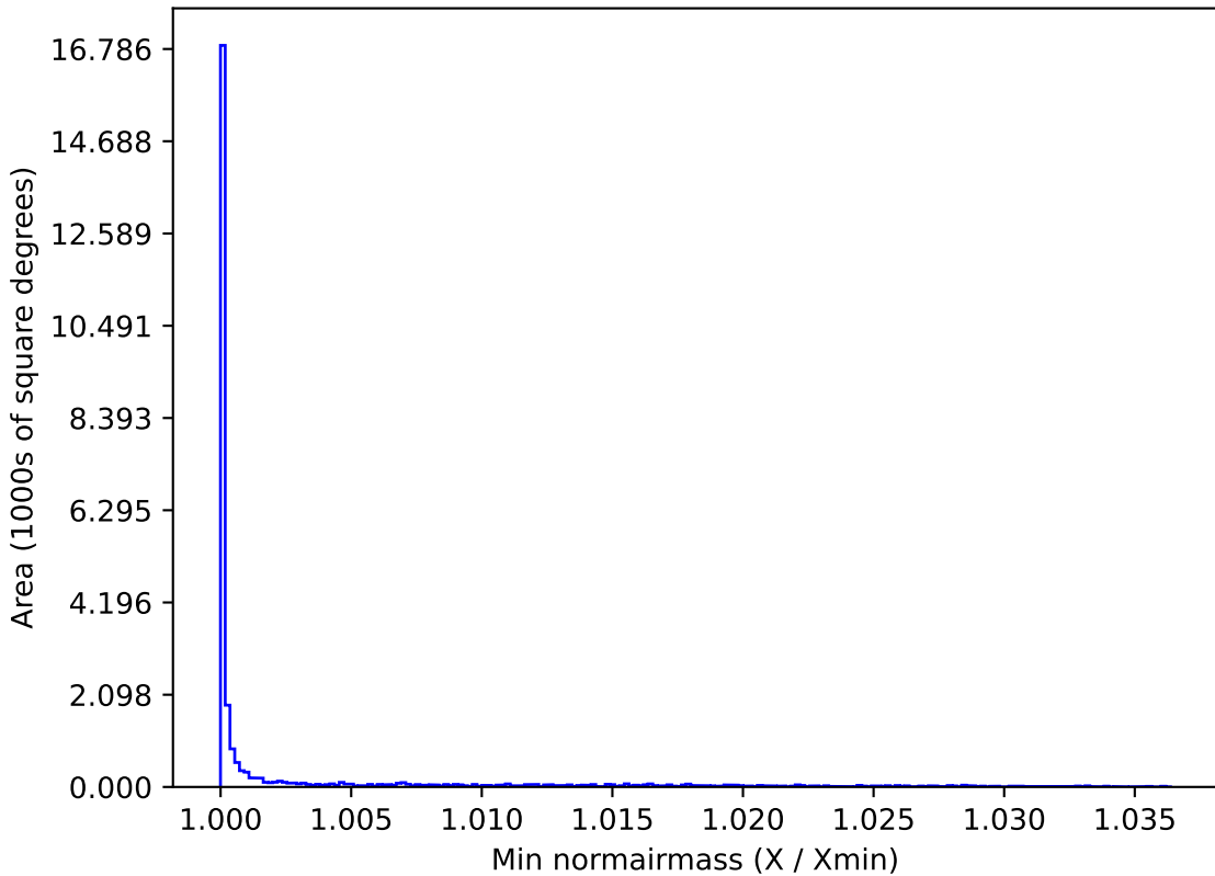
roman_v3.3_10yrs All sky g band: Min normairmass
