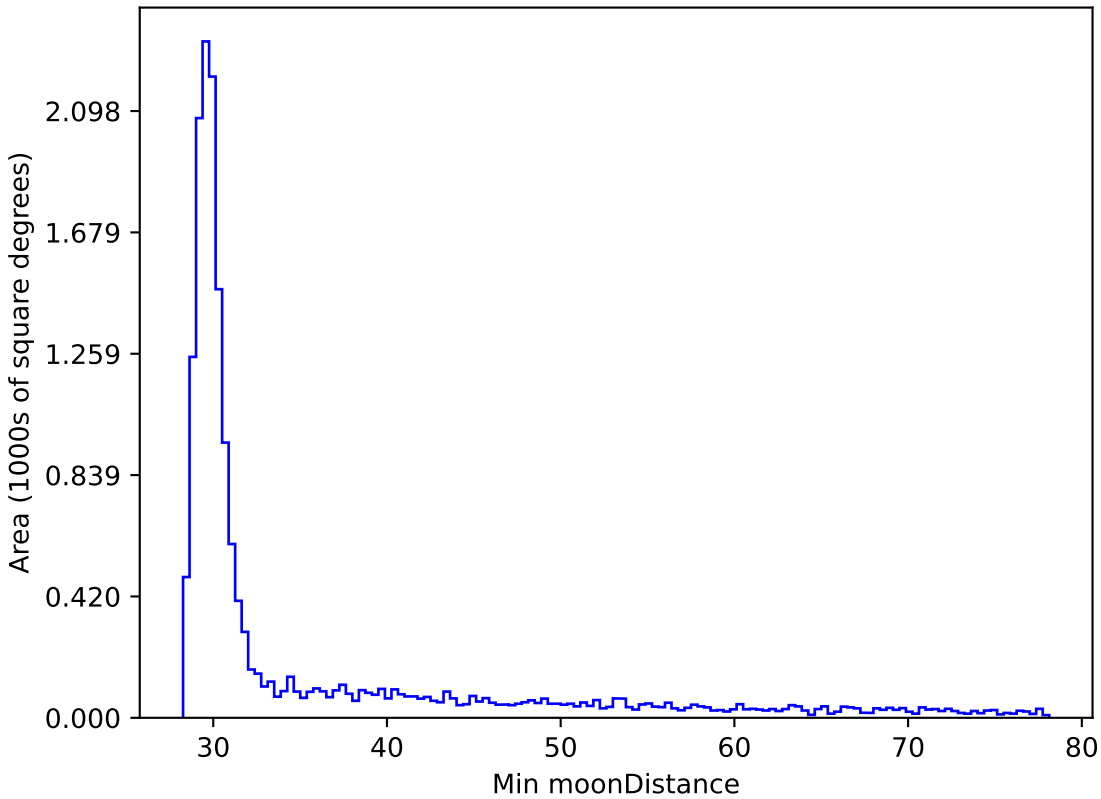
roman_v3.3_10yrs WFD z band: Min moonDistance
