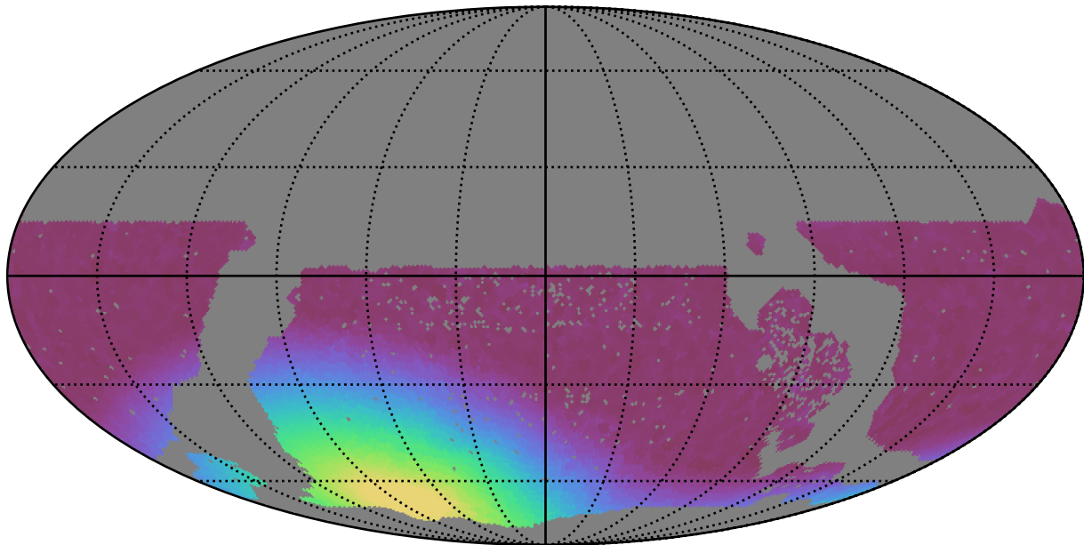
roman_v3.3_10yrs WFD y band: Min moonDistance
