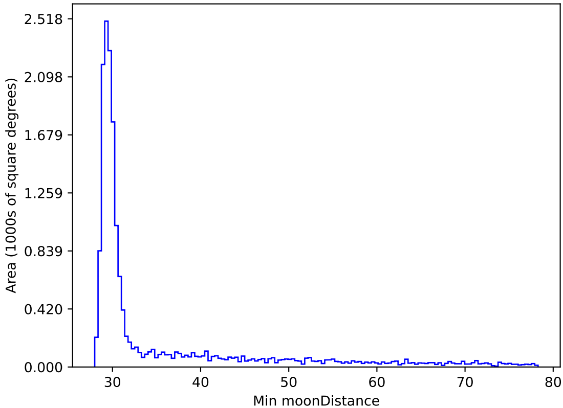
roman_v3.3_10yrs WFD y band: Min moonDistance
