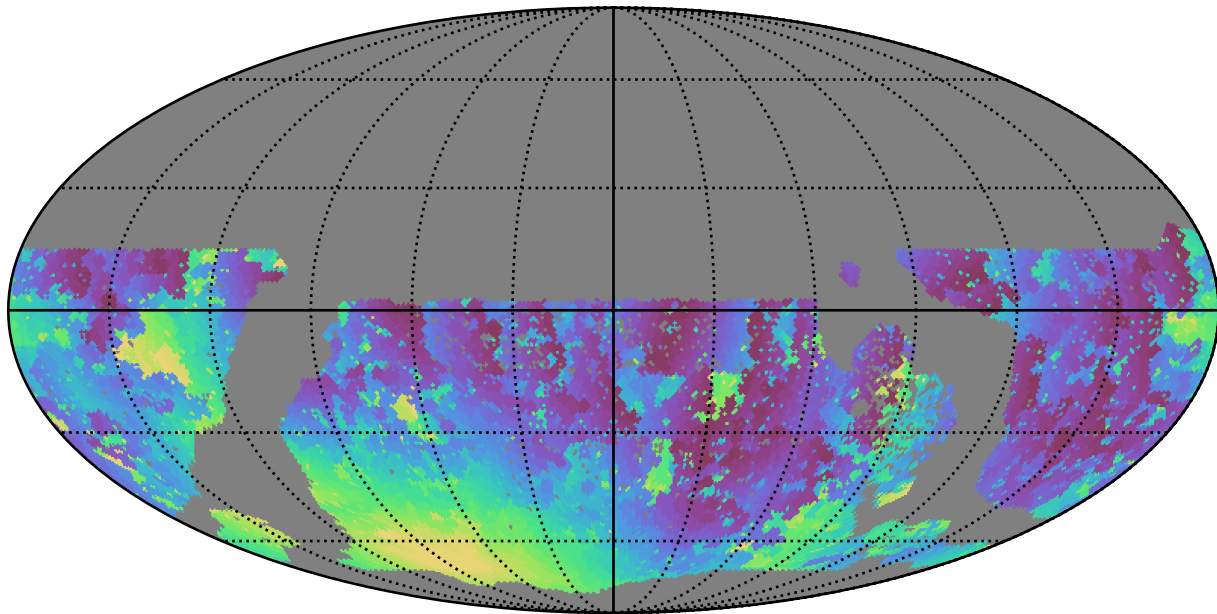
roman_v3.3_10yrs WFD u band: Min moonDistance
